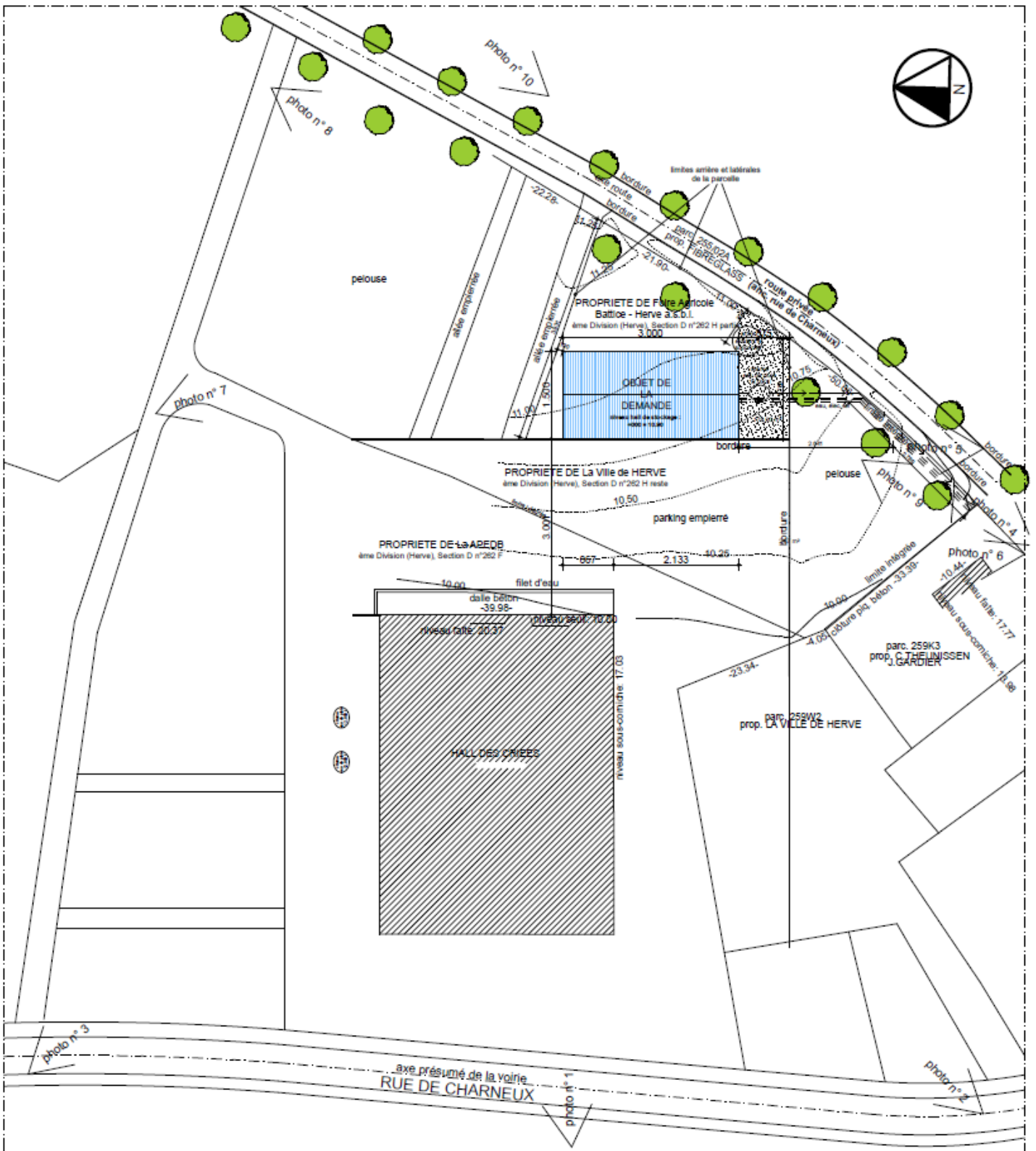
Implantation Echelle 1/500
